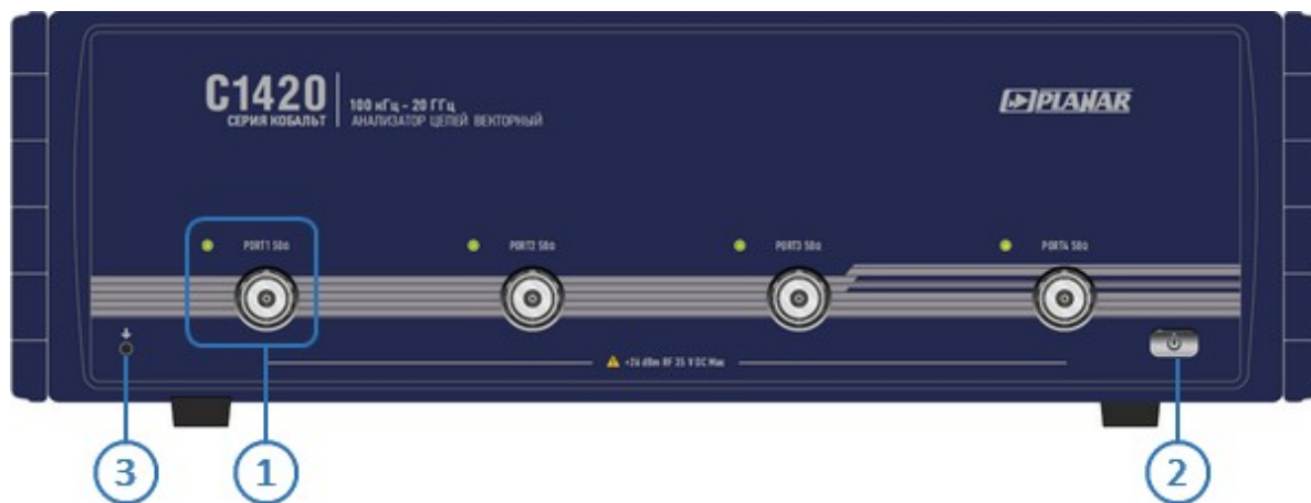
Рисунок 26 – Передняя панель
