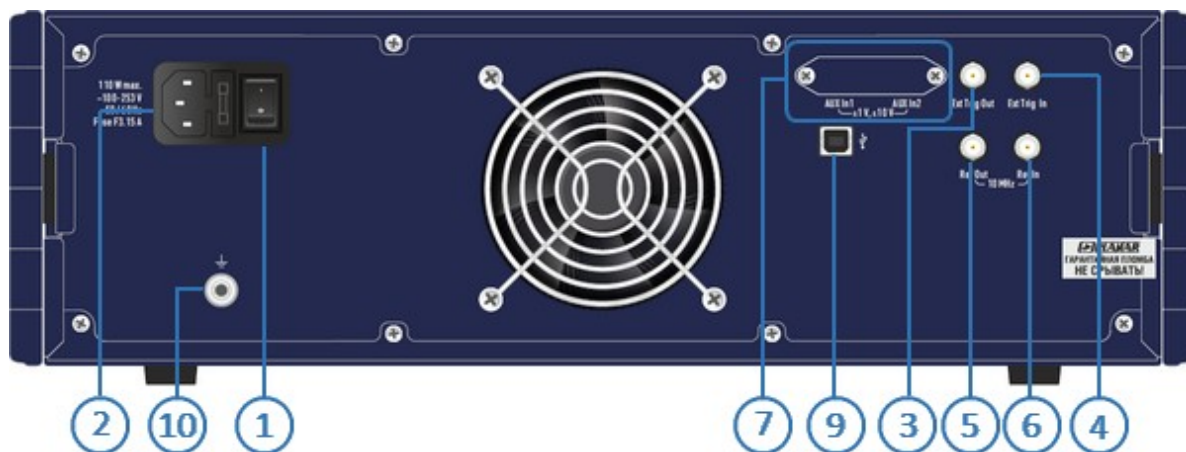
Рисунок 27 – Задняя панель
