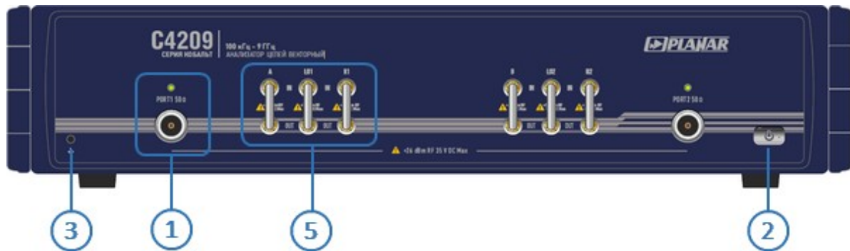
Рисунок 34 – Передняя панель
