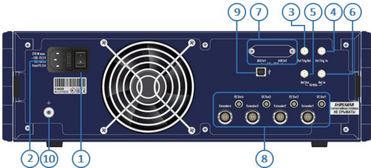
Рисунок 41 – Задняя панель
