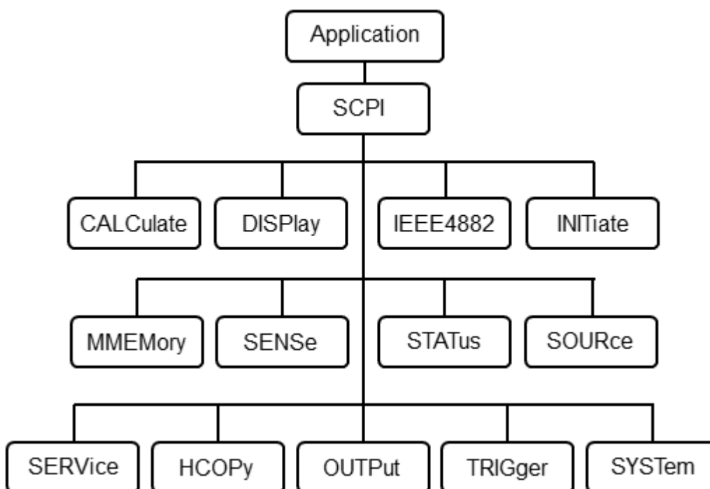
Рисунок 148 –Структура COM-объектов
