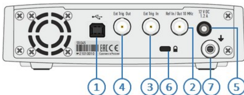
Рисунок 10 – Задняя панель
