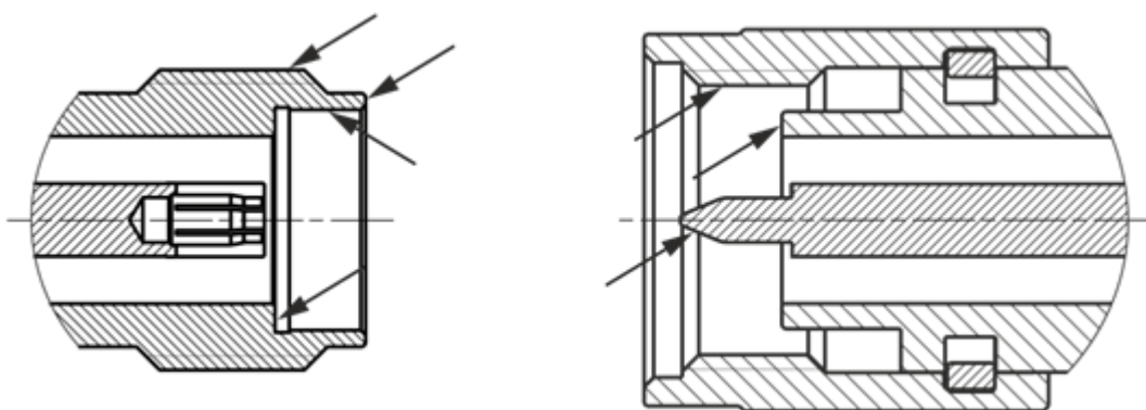
Рисунок 4 – Соединители тип 2,4 мм, 3,5 мм и IX (розетка и вилка)
