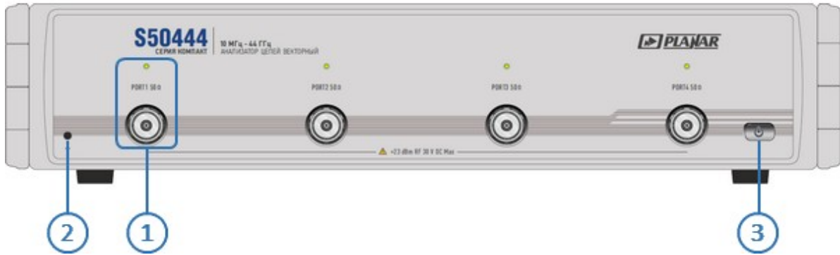
Рисунок 27 – Передняя панель
