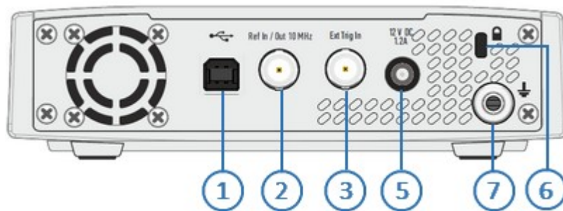
Рисунок 12 – Задняя панель
