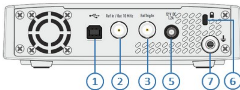
Рисунок 18 – Задняя панель
