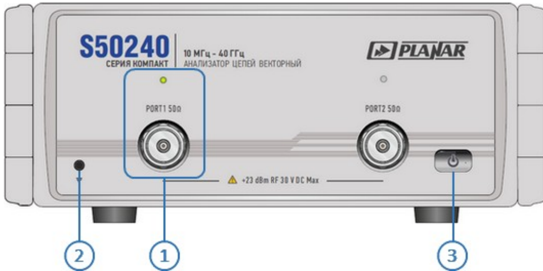
Рисунок 21 – Передняя панель
