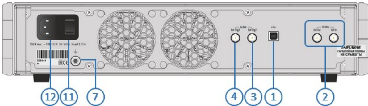
Рисунок 28 – Задняя панель
