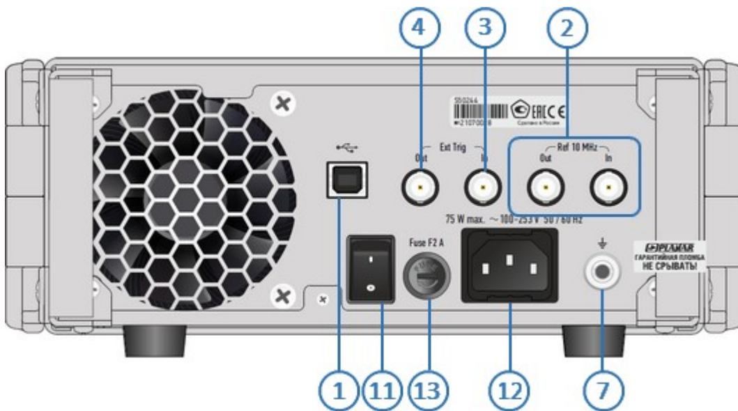
Рисунок 24 – Задняя панель
