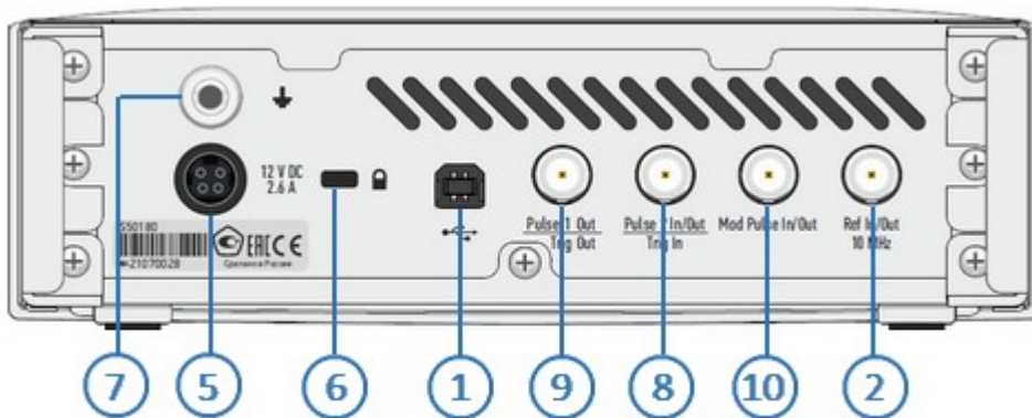
Рисунок 20 – Задняя панель
