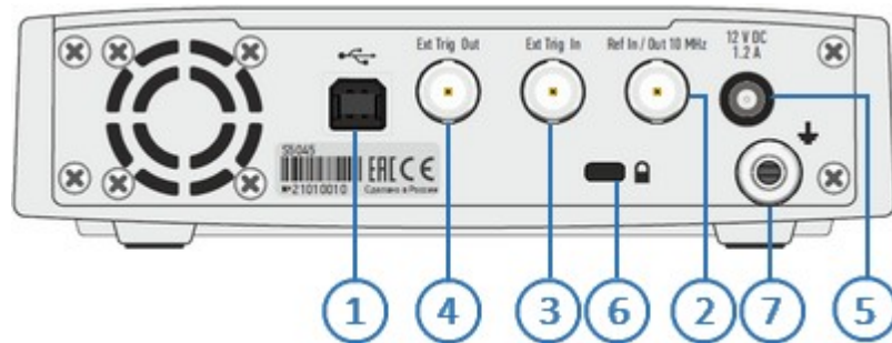
Рисунок 14 – Задняя панель
