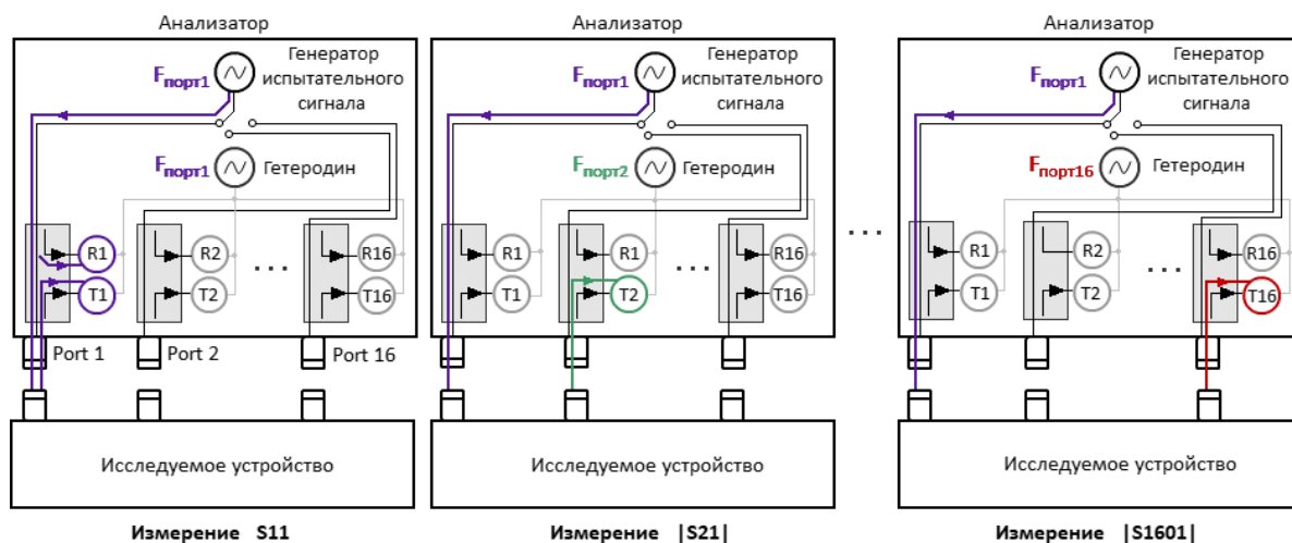
Рисунок 175 — Режим смещения частоты между портами
