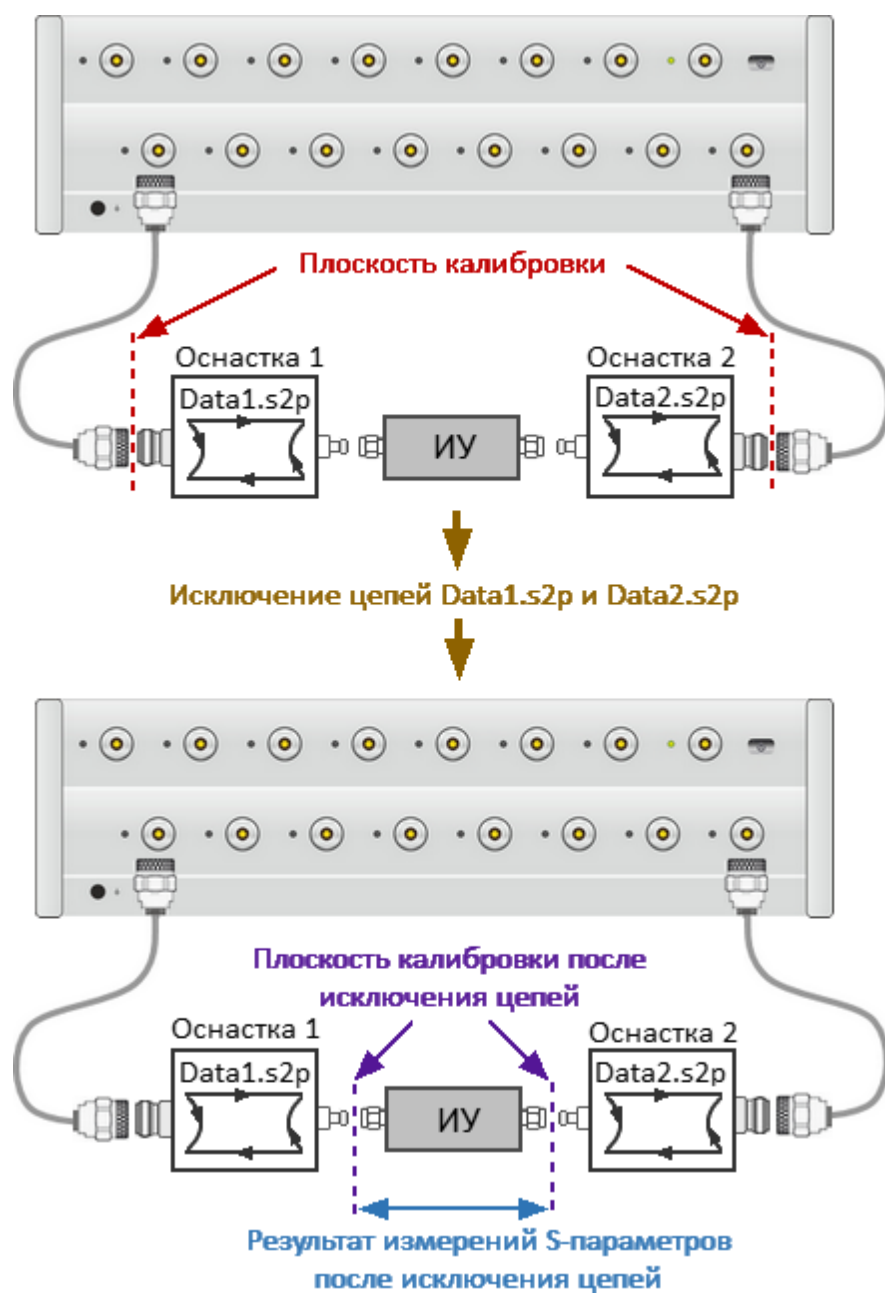
Рисунок 154 — Пример измерения ИУ с исключением цепей
