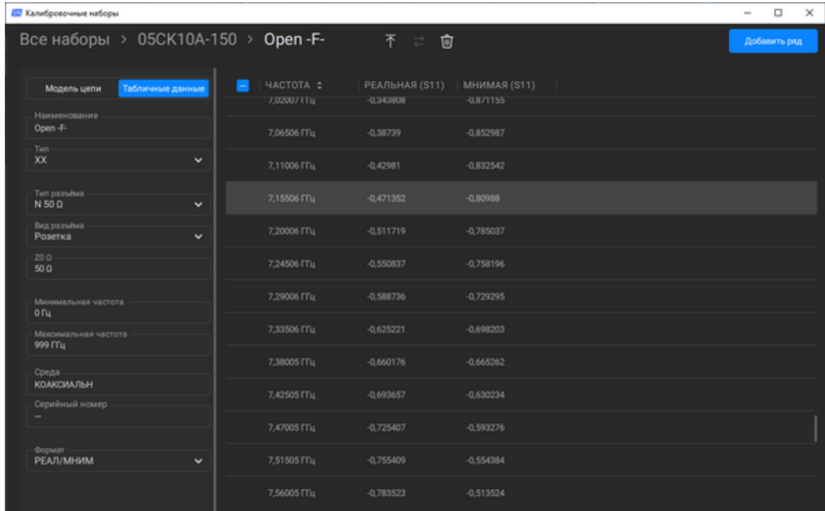
Рисунок 90 — Окно редактирования параметров калибровочной меры, определенной данными
