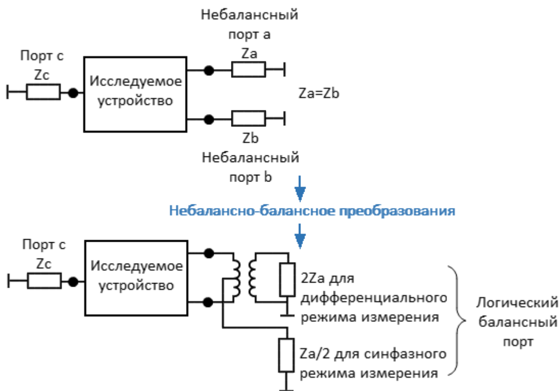
Рисунок 163 — Схема небалансно-балансного преобразования
