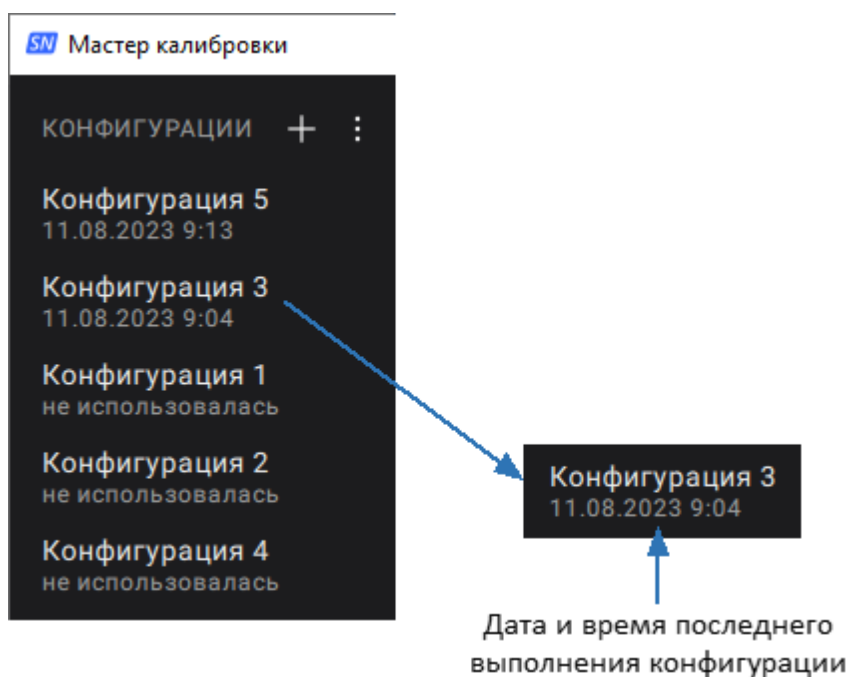
Рисунок 94 — Список конфигураций
