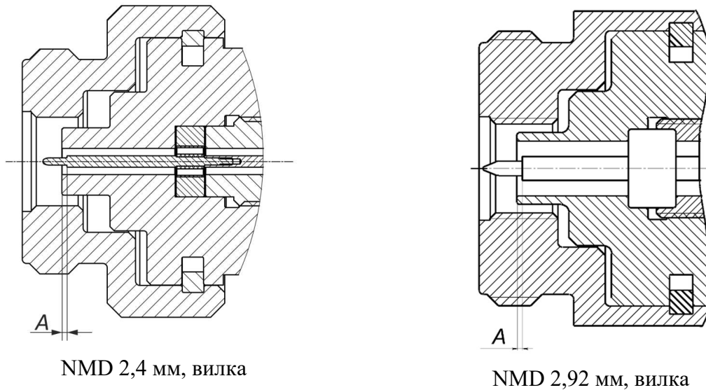
Рисунок А.2 – Присоединительный размер А
