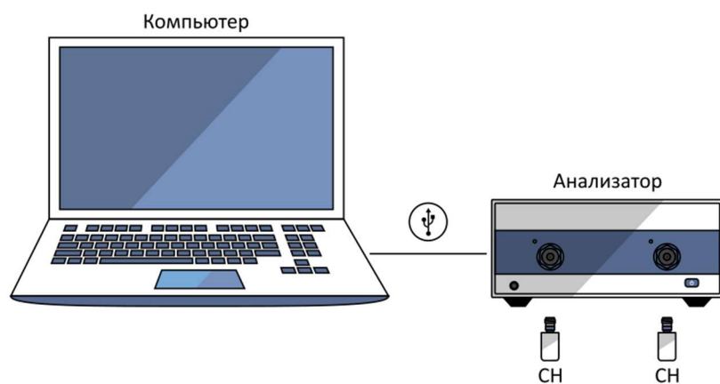
Рисунок А.6 – Схема измерений
